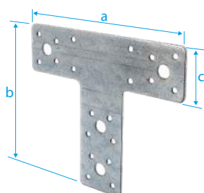
Pletina de ensamble "T", galvanizada Sendzimir
